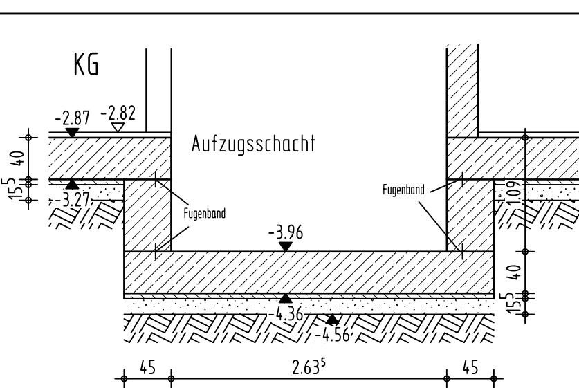
Teilschnitt 1-1
