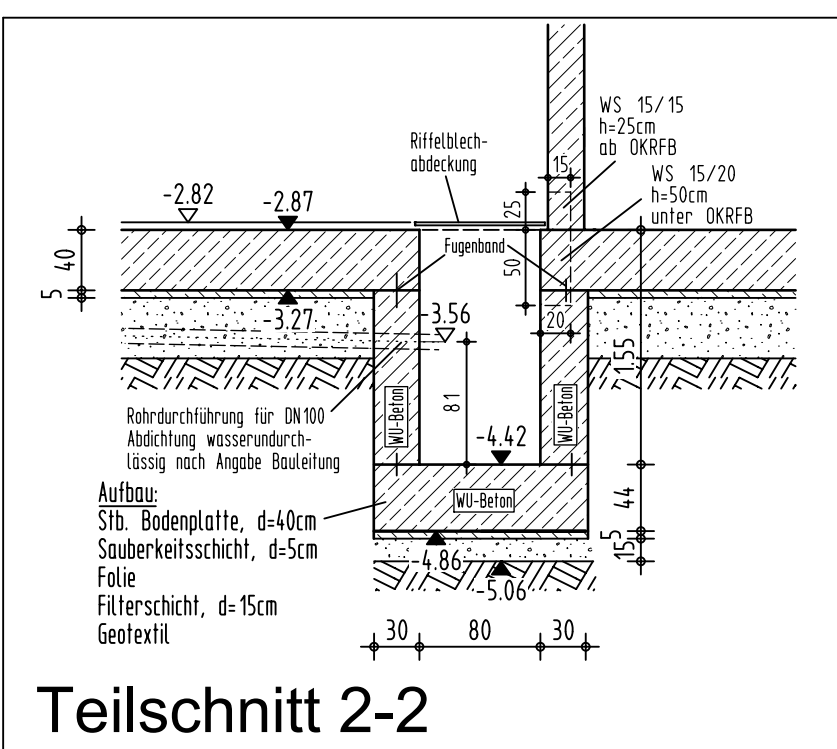
Teilschnitt 2-2
